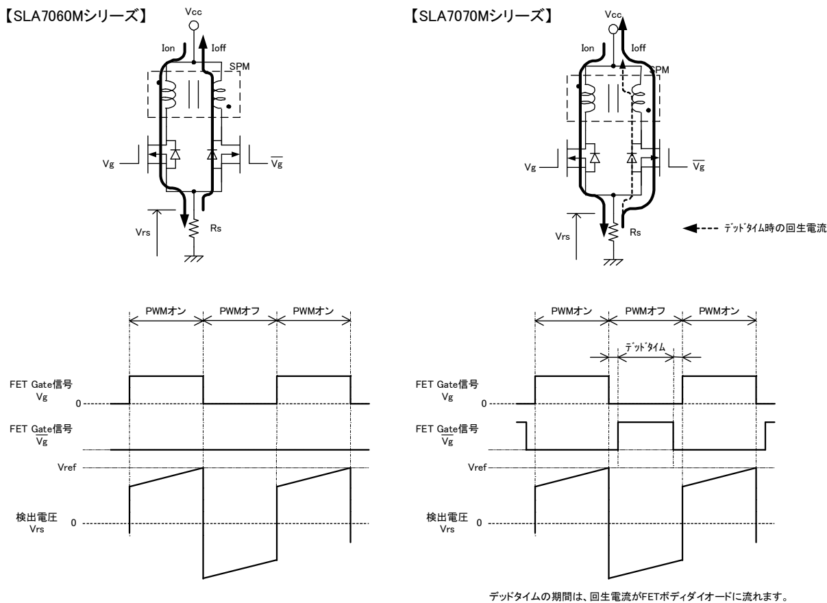
図 14-5 同期整流動作
