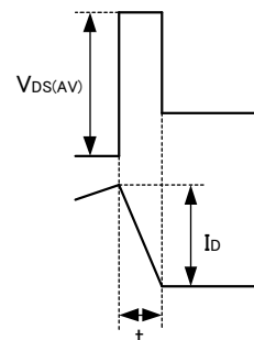
図 15-3 ブレイクダウン時 波形図
