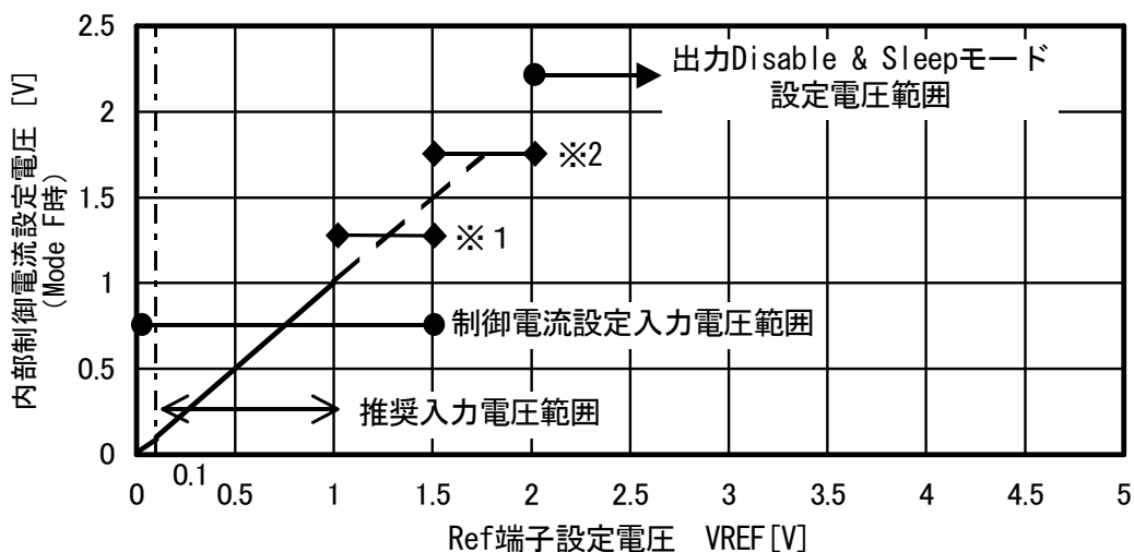
Fig15 - 2 外部-内部 REF 電圧と動作の関係
