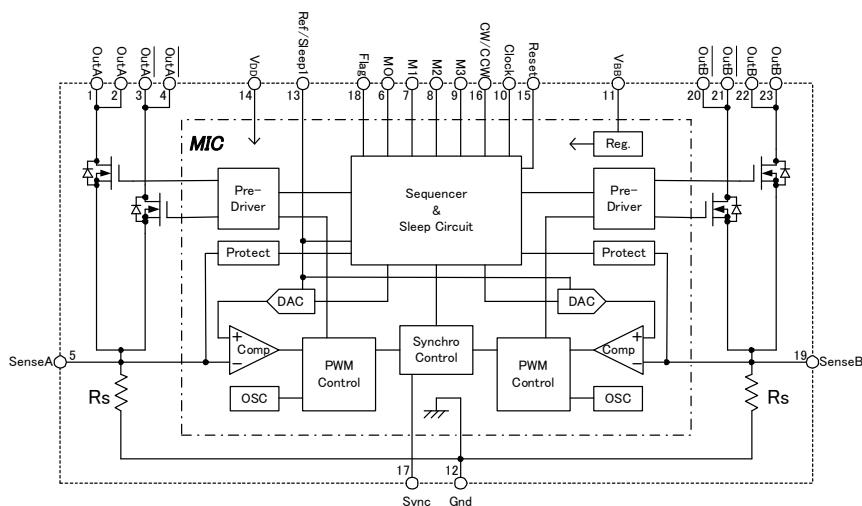
図 7 - 2 SLA7075MPR~SLA7078MPR：μステップ対応品
